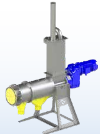
SEPCOM® Horizontal Cow H1-260-3
