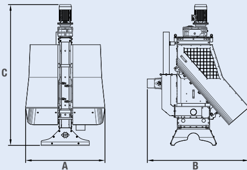
SEPCOM® Vertical Pig V2-150-3
