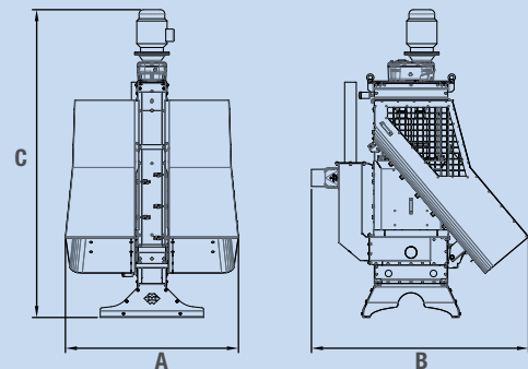
SEPCOM® Vertical Pig V2-200-3
